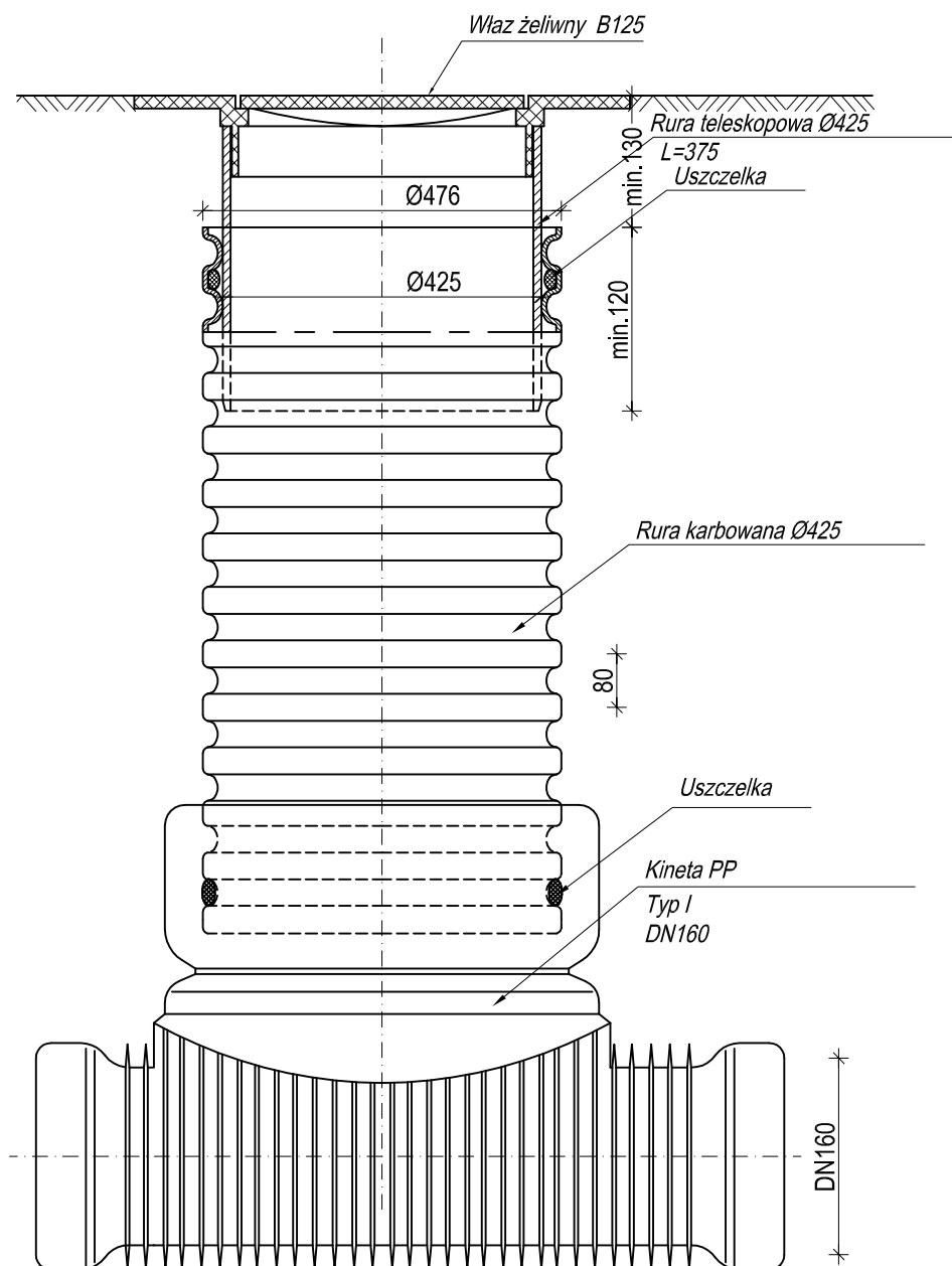
Studzienka rewizyjna Ø425 z rurą teleskopową i włazem żeliwnym typu B125
